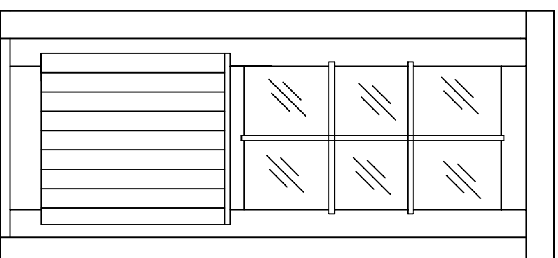
Tür 840x1955
